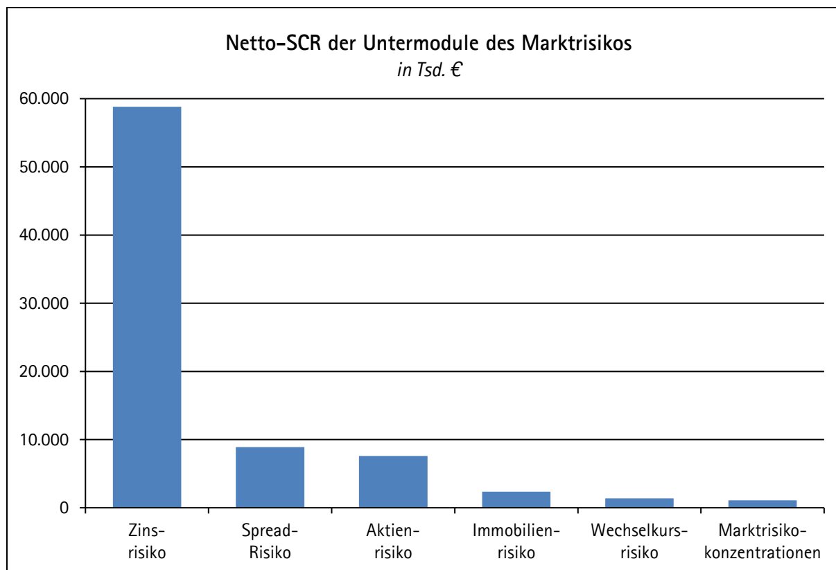
Abbildung 2: Netto-SCR der Untermodule des Marktrisikos
